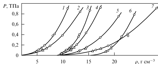
Рис. 5. Ударные адиабаты семи металлов: 1 — Cu ( \rho = 7 \text{ г/см}^3 ); 2 — Cd ( \rho = 7 \text{ г/см}^3 ); 3 — Fe; 4 — Ni; 5 — Sn ( \rho = 2 \text{ г/см}^3 ); 6 — Zn ( \rho = 8 \text{ г/см}^3 ); 7 — Pb ( \rho = 2 \text{ г/см}^3 ); \Delta — [52], \circ — [53].
