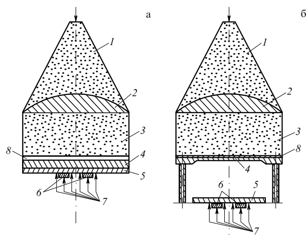
Рис. 3. Контактное взрывное измерительное устройство (а) и взрывное измерительное устройство с разгоном стального ударника (б). 1 — линзовый заряд ВВ; 2 — плосковолновая линза; 3 — основной заряд; 4 — прокладка (а) и ударник (б); 5 — экран из эталонного металла; 6 — исследуемый образец; 7 — электроконтактные датчики; 8 — воздушный зазор (а) и прокладка из плексигласа (б).
