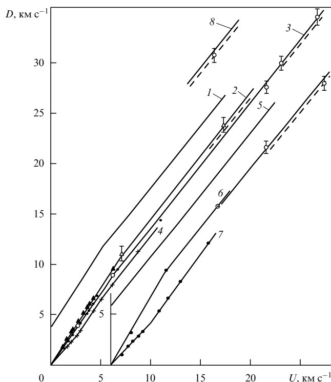
Рис. 16. Зависимости D(U) для пористых железа, меди и вольфрама. 1–4 — адиабаты меди, пористость m = 1, 3, 4, 10 ; 5–7 — адиабаты железа ( u + 6 \text{ км с}^{-1} ), m = 1, 3, 5, 20 ; 8 — адиабата вольфрама, m = 3,1 ; ▲, ●, + — лабораторные измерения; △, ○ — подземные измерения; штриховые линии — расчет по модели ТФПК [177, 178].
