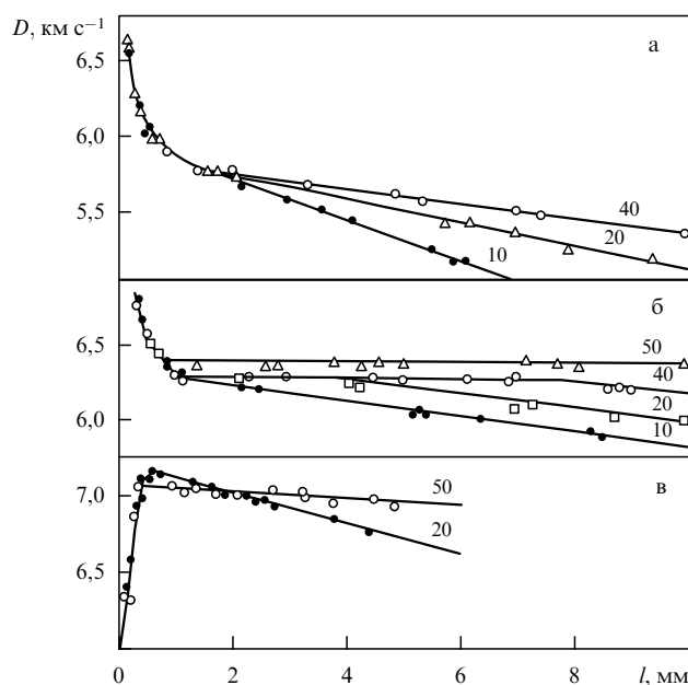
Рис. 2. Изменение скорости ударной волны в плексигласе с расстоянием от зарядов из тротила (а), флегматизированного тэна (б), агатированного гексогена (в). Цифры у кривых отвечают длине заряда в мм.
