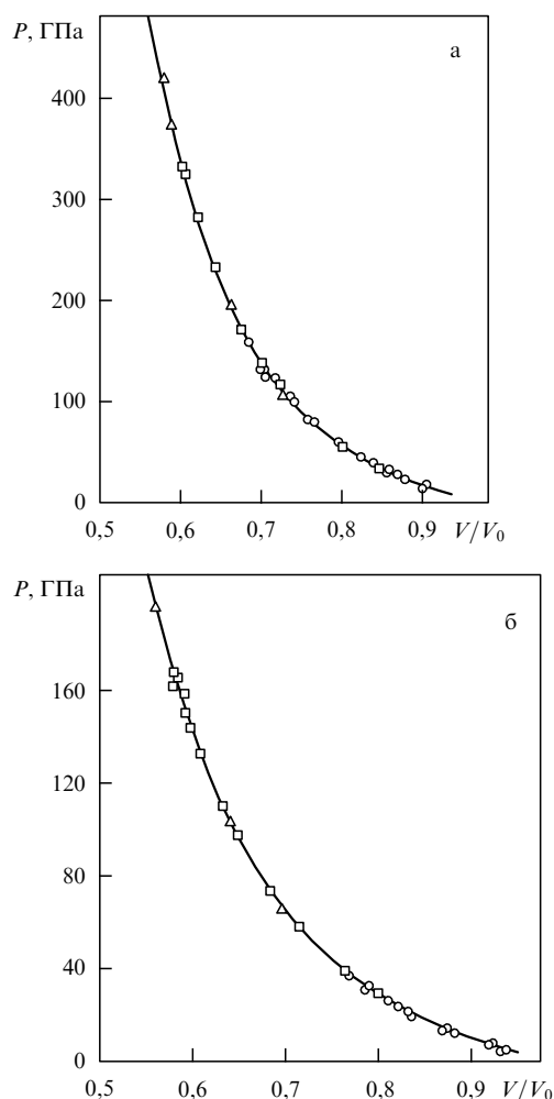
Рис. 6. Ударные адиабаты меди (а) и алюминия (б). Данные измерений на взрывных устройствах: \triangle — [51], \circ — [52, 60], \square — данные измерений на легкогазовой пушке [61]. V_0 — начальный объем.
