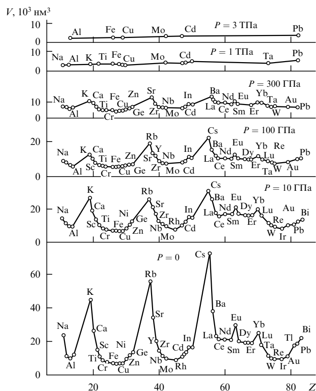
Рис. 8. Кривые атомных объемов V(Z) для нормальных условий ( P = 0 ) и различных уровней ударного сжатия.
