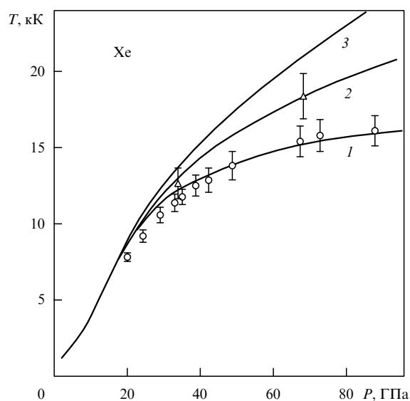
Рис. 20. Зависимость яркостной температуры фронта ударной волны в ксеноне от давления. Экспериментальные данные: ○ — \lambda = 0,67 мкм [232], △ — \lambda = 0,32 мкм [233]. Расчет: 1, 2 — яркостные температуры для \lambda = 0,67 и 0,32 мкм соответственно [232], 3 — равновесная температура.
