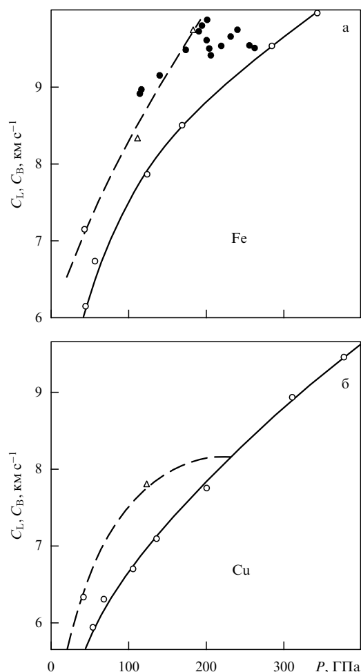
Рис. 12. Зависимости продольной C_L (штриховая линия) и объемной C_B (сплошная линия) скорости звука в железе (а) и меди (б) по данным \circ — [141], \triangle — [143], \bullet — [144].
