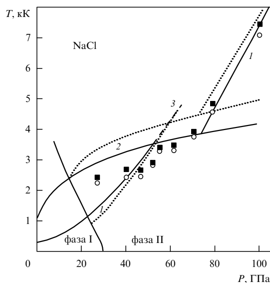
Рис. 19. Фазовая диаграмма хлористого натрия. ■, ○ — экспериментальные значения температур в области спектра \lambda = 0,478 и 0,625 мкм соответственно, 1 — ударная адиабата, 2 — кривая плавления, 3 — ударная адиабата "перегретой" твердой фазы; сплошные линии — расчет для фазы I, пунктир — для фазы II.
