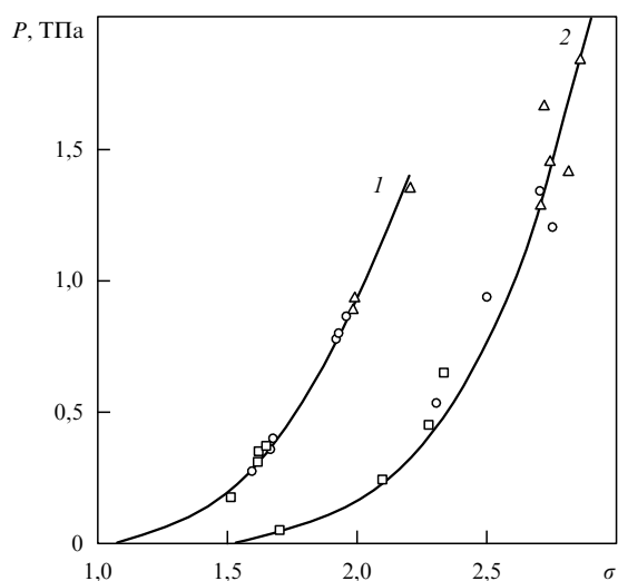
Рис. 7. Ударные адиабаты: 1 — железа и 2 — урана ( \sigma + 0,5 ). \circ — данные измерений на однокаскадных устройствах, \triangle — данные измерений на двухкаскадных устройствах, \square — данные [62]. Относительная плотность \sigma = \rho/\rho_0 .
