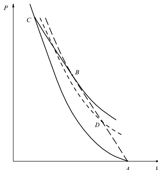
Рис. 1. P – V диаграмма стационарной детонации. A – C — ударная адиабата, B — точка Жуге, B – C — зона реакции, D — состояние недетонировавшего ВВ.
