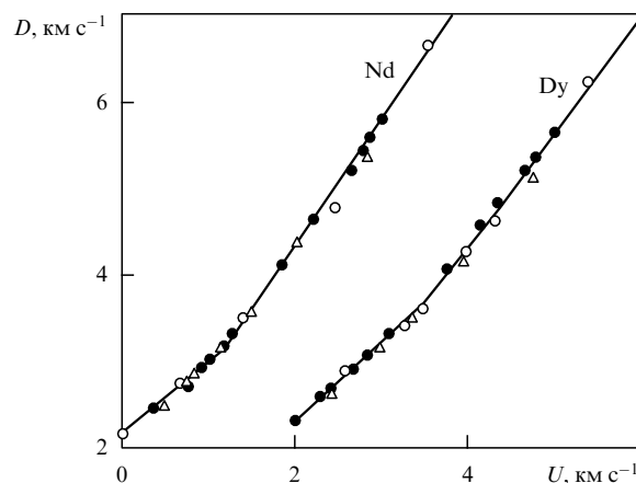
Рис. 10. Зависимости D(U) для Nd и Dy ( U + 2 км с -1 ): \circ — данные [75], \triangle — данные [78], \bullet — данные [79].
