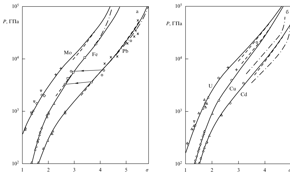
Рис. 13. Результаты лабораторных и подземных измерений ударного сжатия молибдена ( \sigma = 0,6 ), железа и свинца (а) и урана ( \sigma = 0,5 ), меди и кадмия (б). \triangle — лабораторные измерения [66], \nabla — лабораторные измерения [55]. Измерения в подземных испытаниях: \square — абсолютные измерения [88], \diamond — абсолютные измерения [95], \circ — относительные измерения [66, 169, 174], + — относительные измерения [182–185], \times — относительные измерения [180]. Штриховые линии — расчет по модели ТФПК [182, 185], штрихпунктир — расчет по модели ССП [264].
