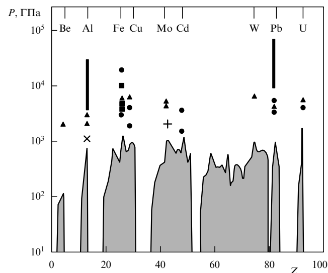
Рис. 14. Диапазоны абсолютных и относительных измерений, достигнутые в лабораторных и подземных испытаниях. Затененная зона отвечает абсолютным лабораторным измерениям, ■, • — абсолютные и относительные подземные измерения ВНИИЭФ; ×, | — то же, ВНИИТФ; +, ▲ — то же, американские данные.
